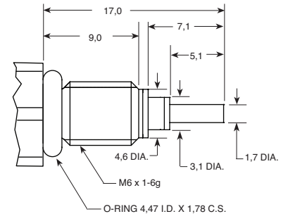
TTS-X-235(M)
