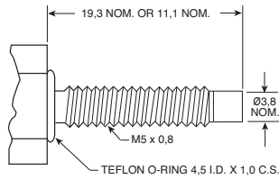
CTL-190M M5X0,8
